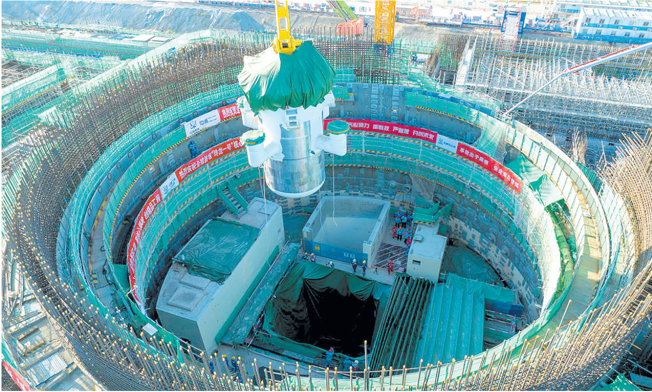
“玲龙之心”安装现场。8月10日,海南省昌江核电站“玲龙一号”全球首堆核心模块安装成功。
