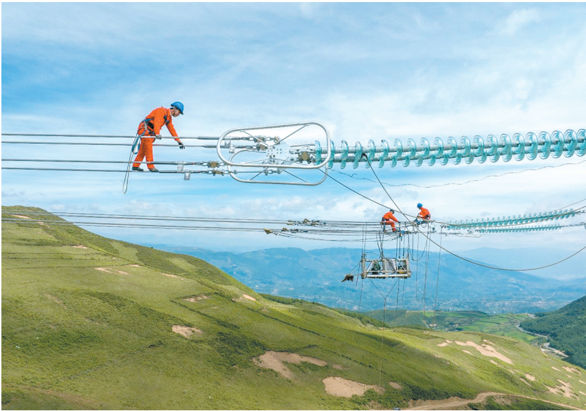
500千伏建叙线施工现场
