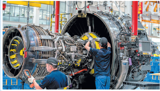
尖端维护 民航喷气发动机维护 (刘婷 摄于成都双流国际机场)
